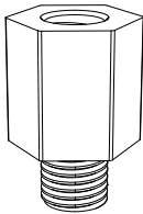
六角螺栓 外#6-32 / 内M3 x3 主板固定
